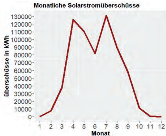
Monatliche Solarstromüberschüsse mit der aktuell installierten Leistung
